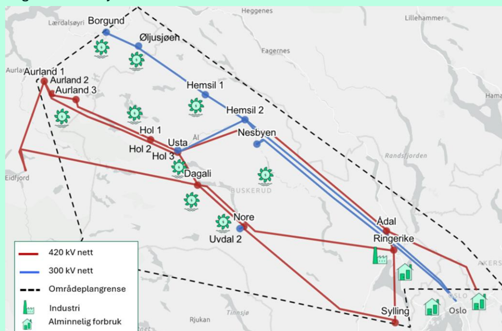
Dagens transmisjonsnett
